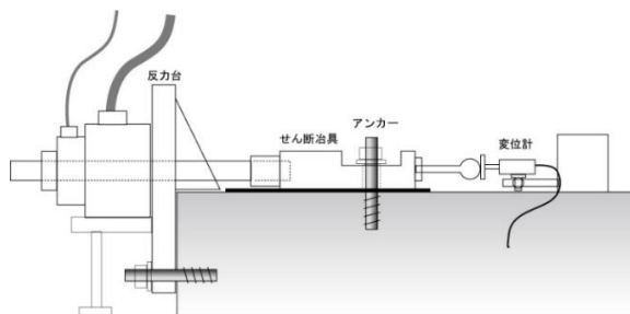
図10: 試験体構成イメージ
