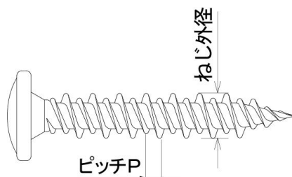
図1. ねじ概要
