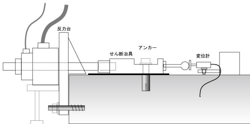
図11: 試験体構成イメージ
