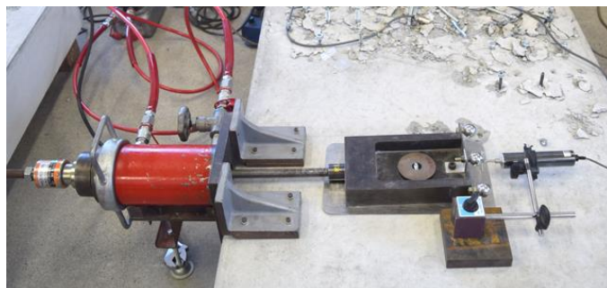
図12: 試験体構成イメージ
