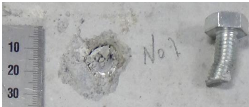
図14: 破壊形態典型
