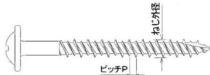
図1. ねじ概要
