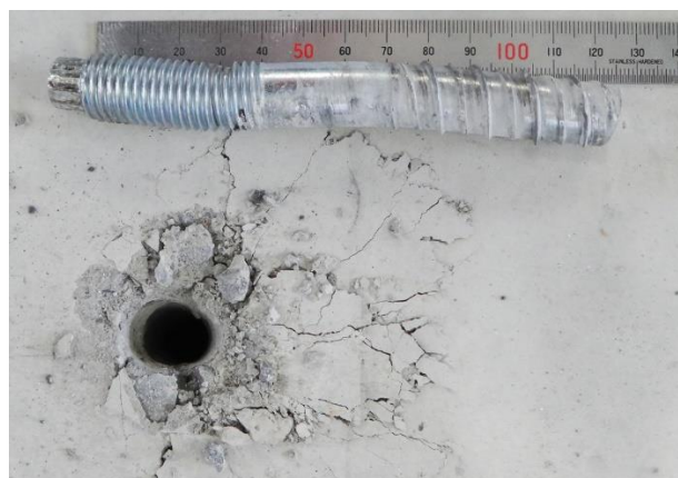
図13:破壊形態 (No3) コンクリートの支圧破壊
