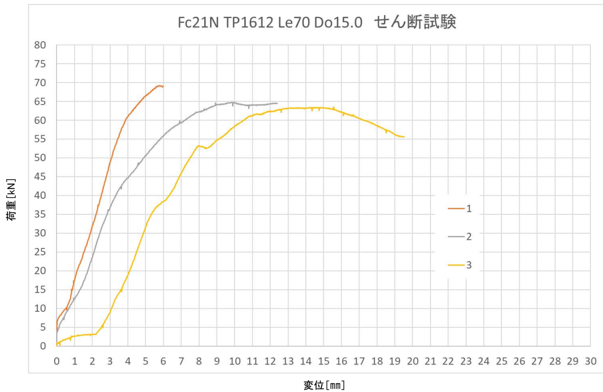
図11:荷重変位曲線
