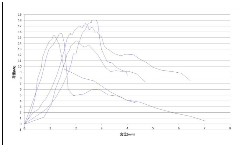
図11:荷重変位曲線
