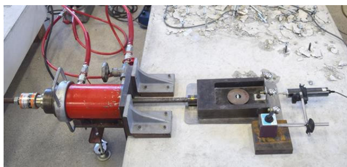
図11: 試験状態
