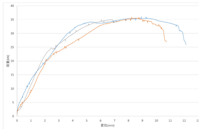
図12: 荷重変位曲線
